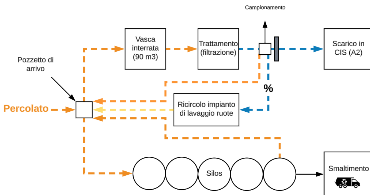
Impianto di trattamento del percolato
